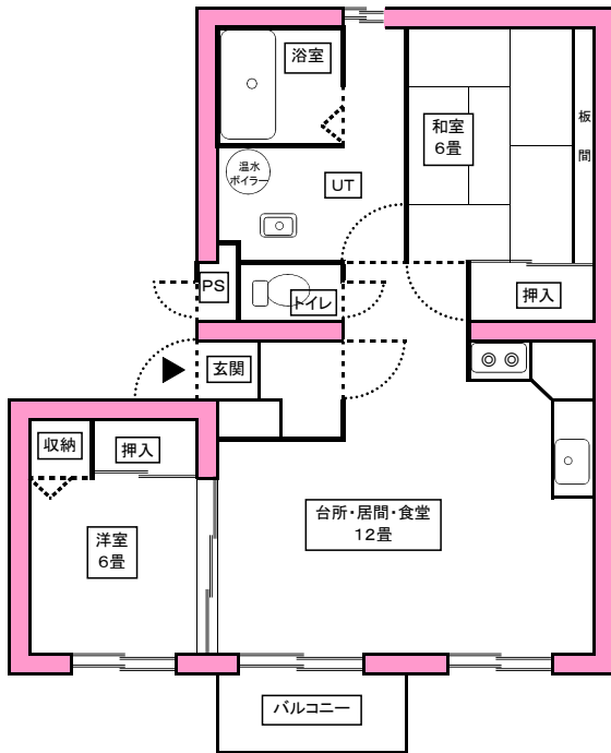
2DK-A (63.80㎡)
