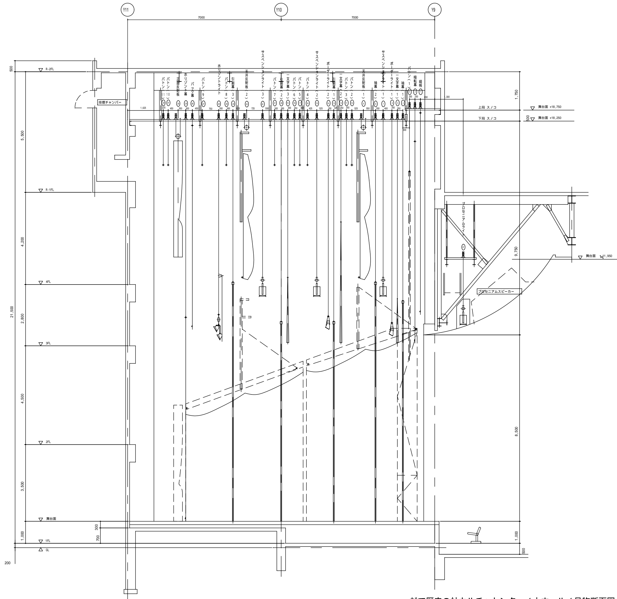
だて歴史の杜カルチャセンター / 大ホール / 吊物断面図 / S = 1 / 100
