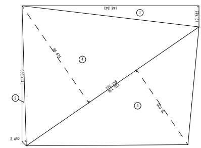
敷地面積求積図 1/2000
